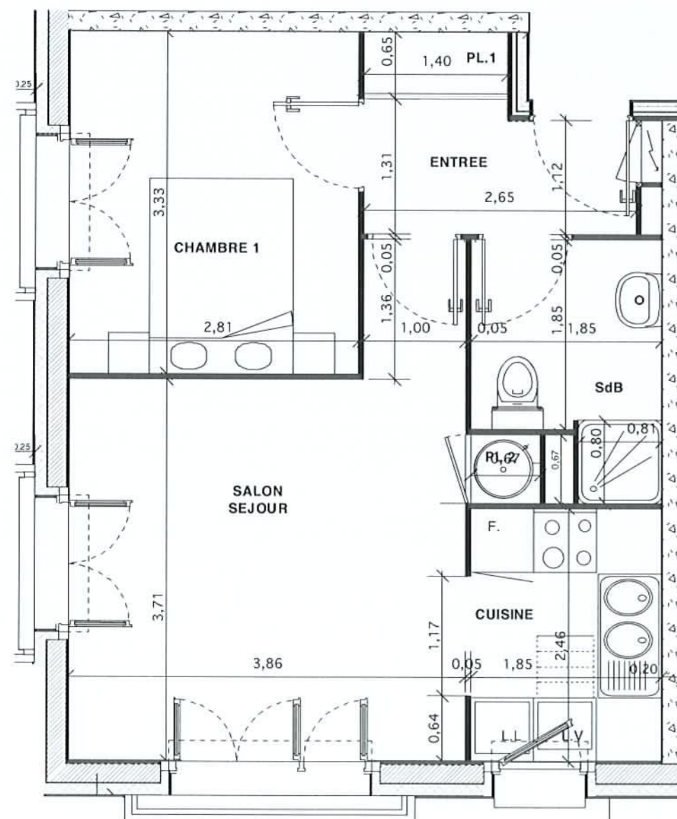
PLAN - éch.1/50
